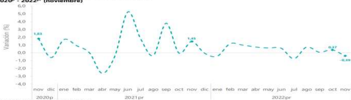
Gráfico 16. Tasa de crecimiento mensual del índice de las actividades terciarias Serie ajustada por efecto estacional y calendario 2020 p - 2022 pr (noviembre)
