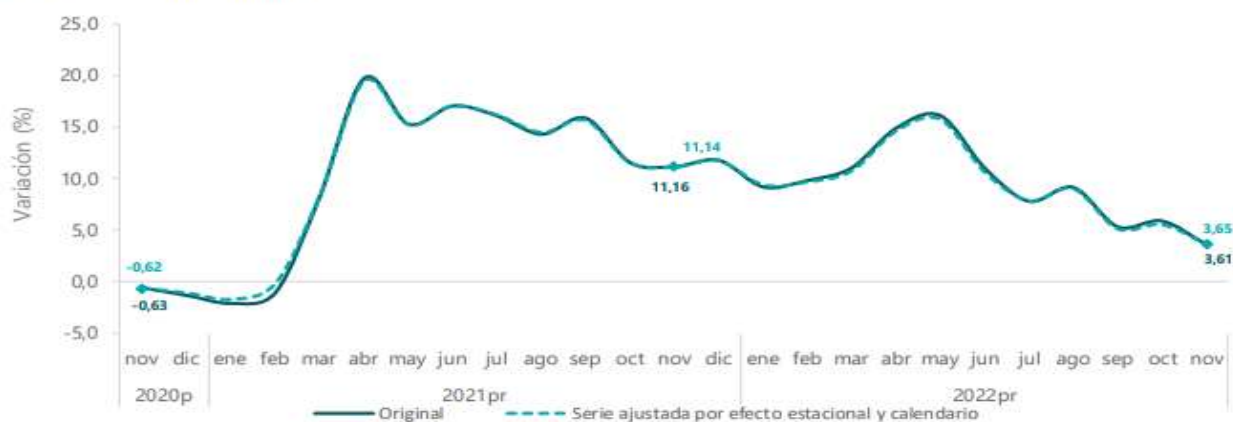
Gráfico 15. Tasa de crecimiento anual del índice de las actividades terciarias Serie original y serie ajustada por efecto estacional y calendario 2020 p - 2022 pr (noviembre)
